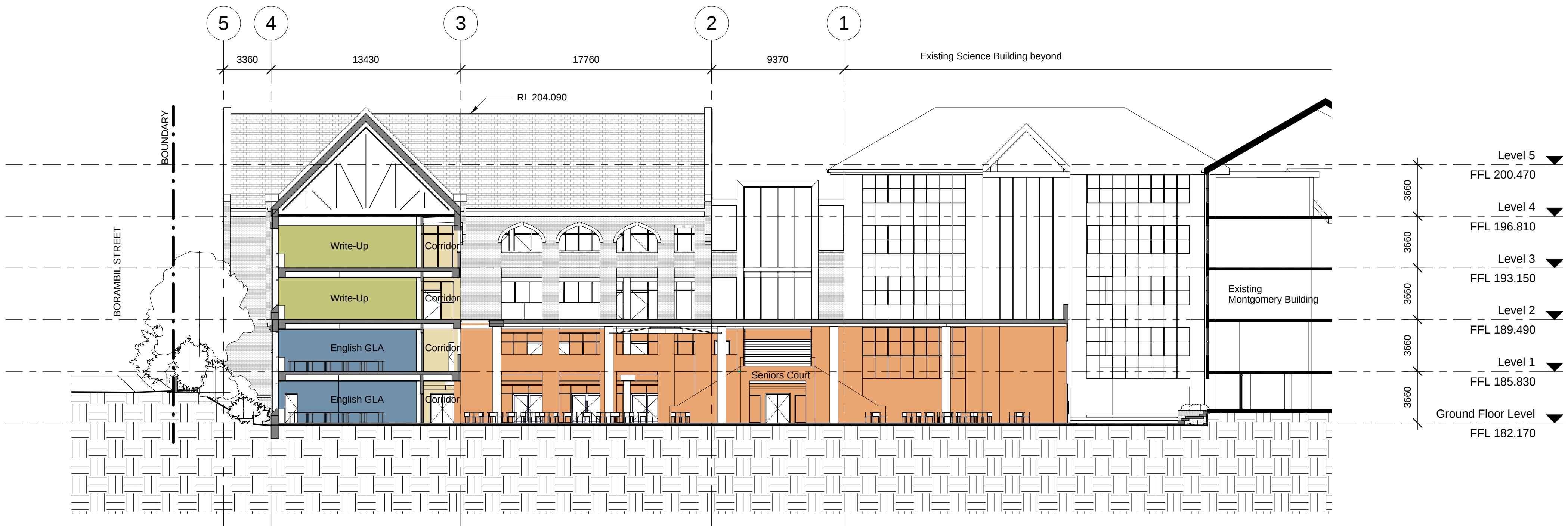
D Section D - D 1 : 200
