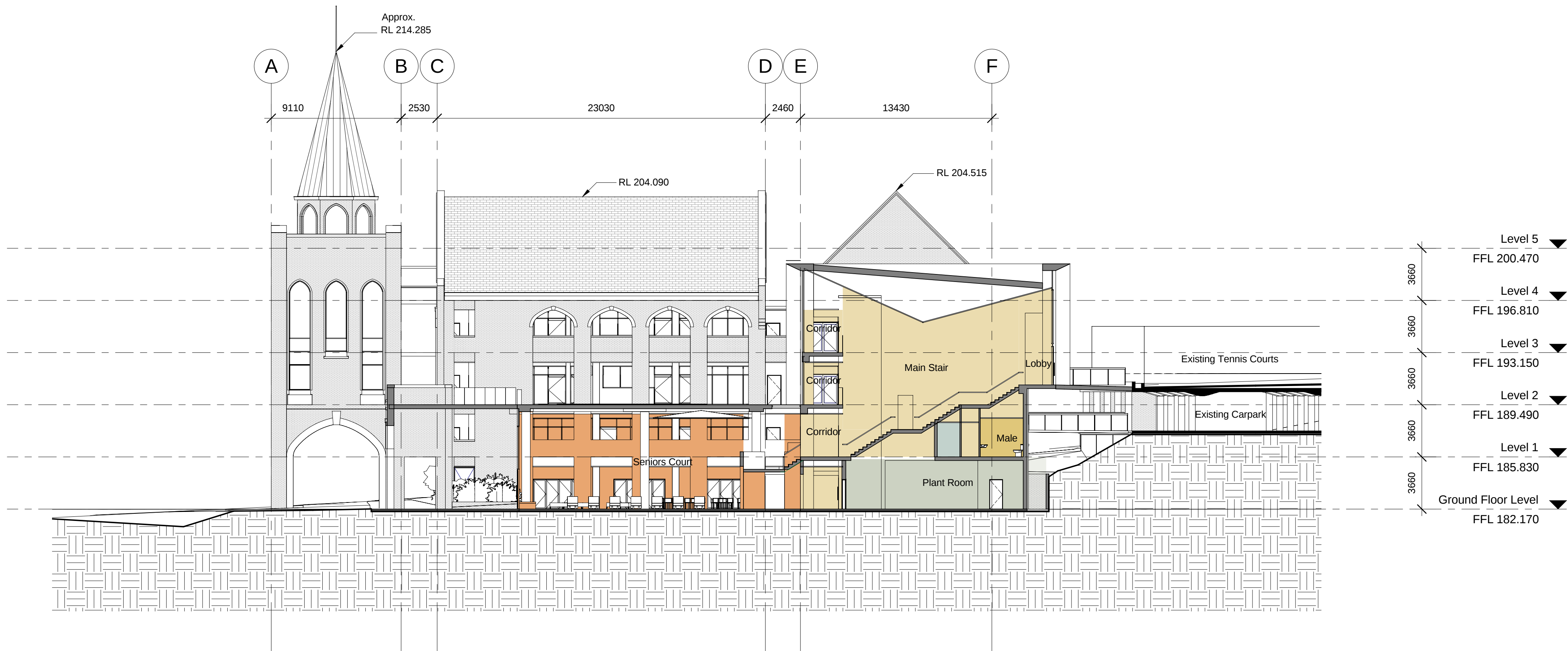
C Section C - C 1 : 200
